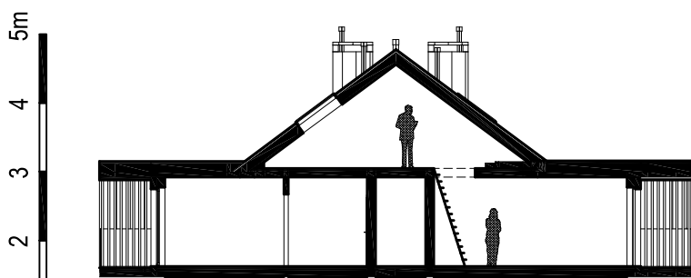
PRZEKRÓJ
