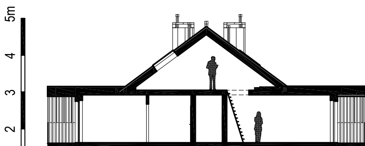
PRZEKRÓJ
